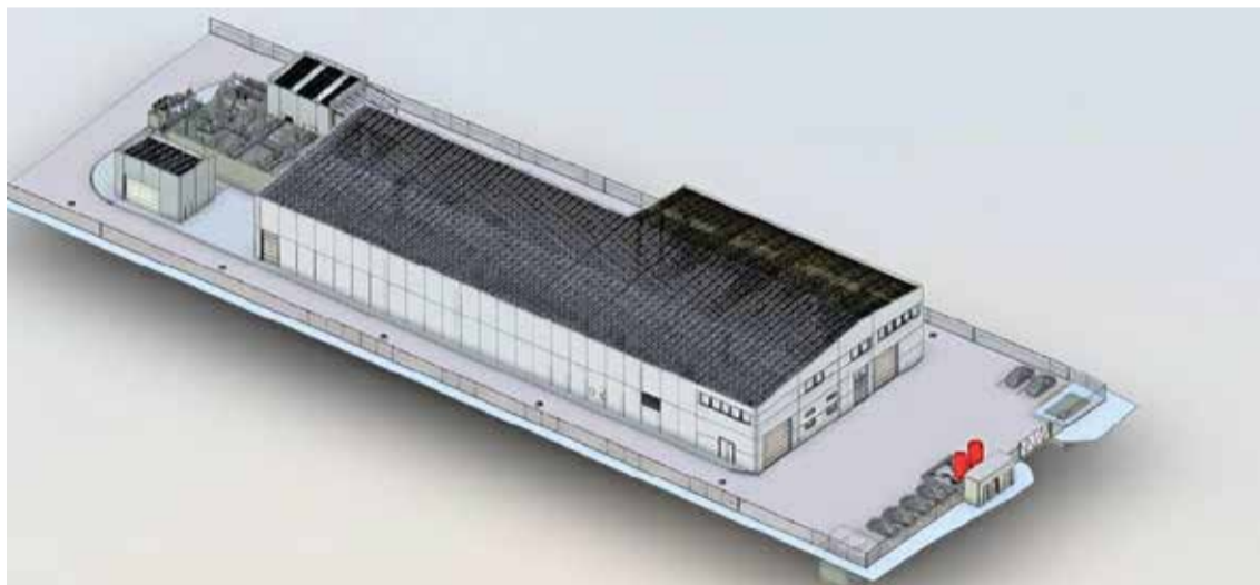
L'EDIFICI PRINCIPAL. Allotjarà espais com el decantador, zona de treball, filtres, dipòsits, aigua, desinfecció i sales de clor
